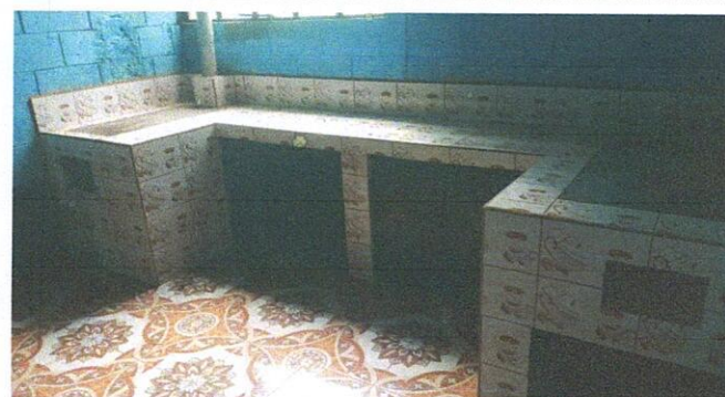
Foto 10: planchas de metal y chimenea, colocacion de azulejos en los polletones y en el piso de la cocina, colocacion de compartimiento puertas de metal.
